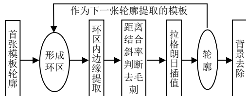
图1 基于模板参照的背景去除流程图
