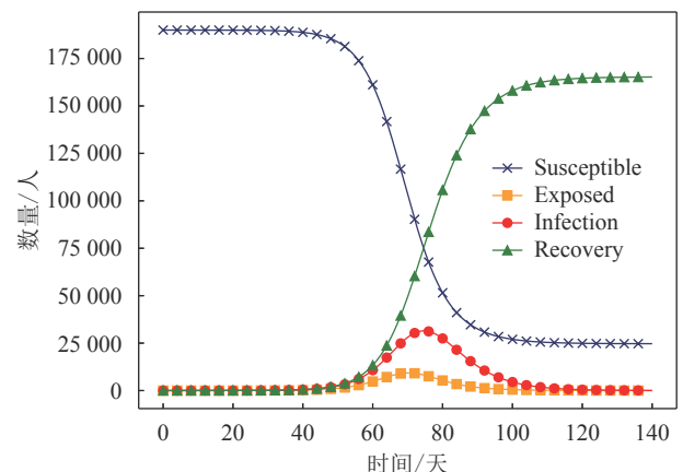
图4 基于 SEIR 模型的仿真结果 (潜伏期 7 天)
