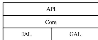
图1 嵌入式GUI分层结构图
