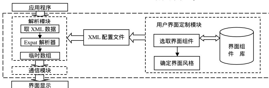
图1 基于XML的可定制界面管理机制图
