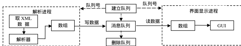
图4 进程间通信原理示意图
