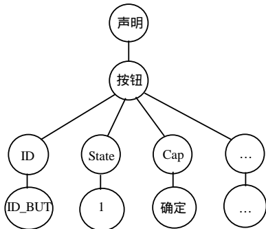
图6 DOM树
