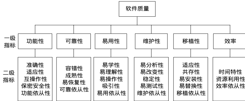
图1 软件质量评估体系
