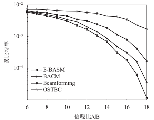
图 5 信道相关性对性能的影响
