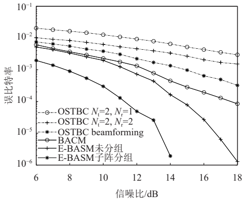
图 3 不同方案性能对比
