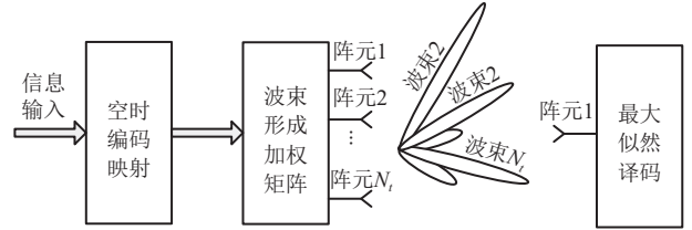
图 1 特征波束赋形传输
