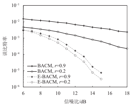
图 6 道相关性对性能的影响
