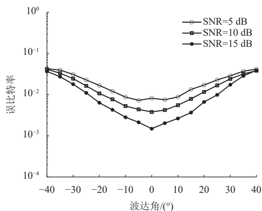
图 7 波达角对不同传播路径译码性能的影响
