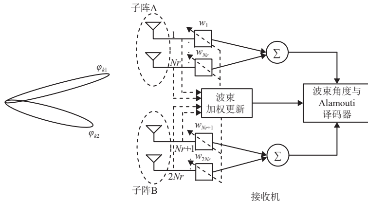
图2 接收机天线分组接收框图
